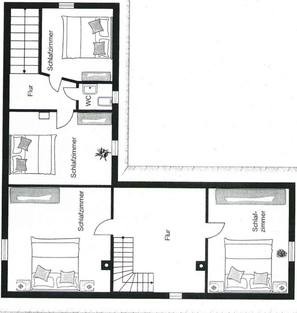
Dachgeschoss
