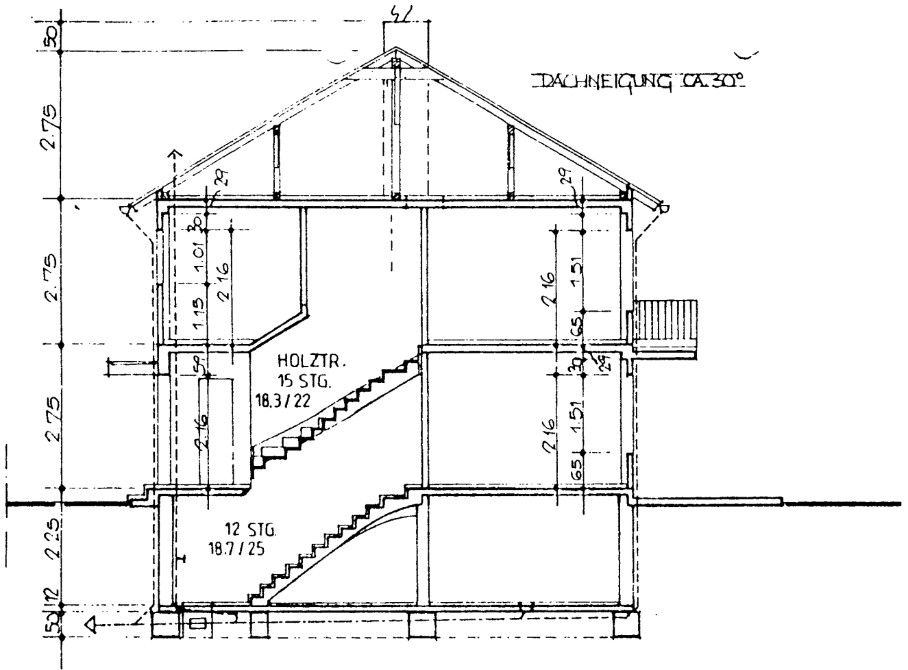
SCHNITT 1-1
