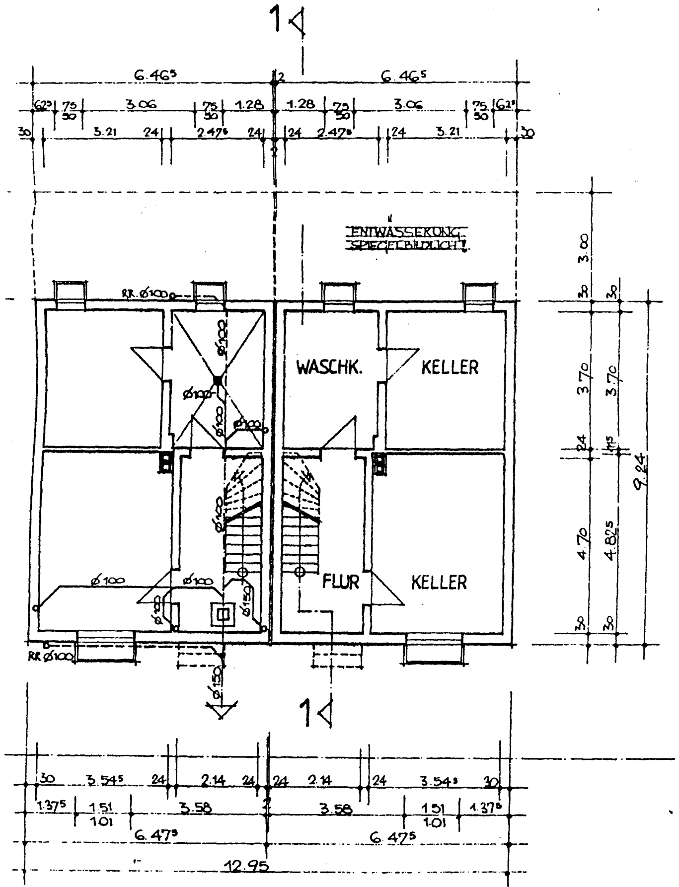
KELLERGESCHOSS
